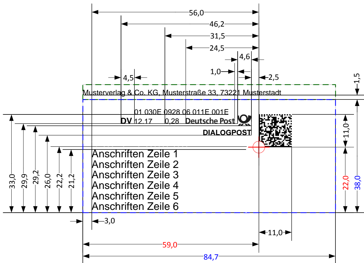
Abbildung 3: Maßzeichnung Adressfenster
